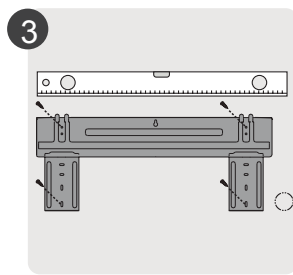
Закрепите монтажную пластину внутреннего блока
