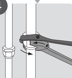
Соединение труб хладагента
