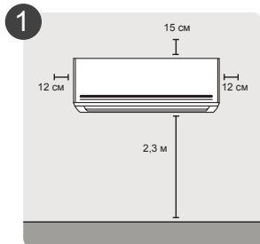
Выберите место монтажа внутреннего блока
