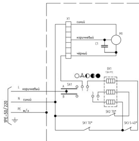
Рис. 3 Электрическая схема завесы КЭВ-5П1141Е
