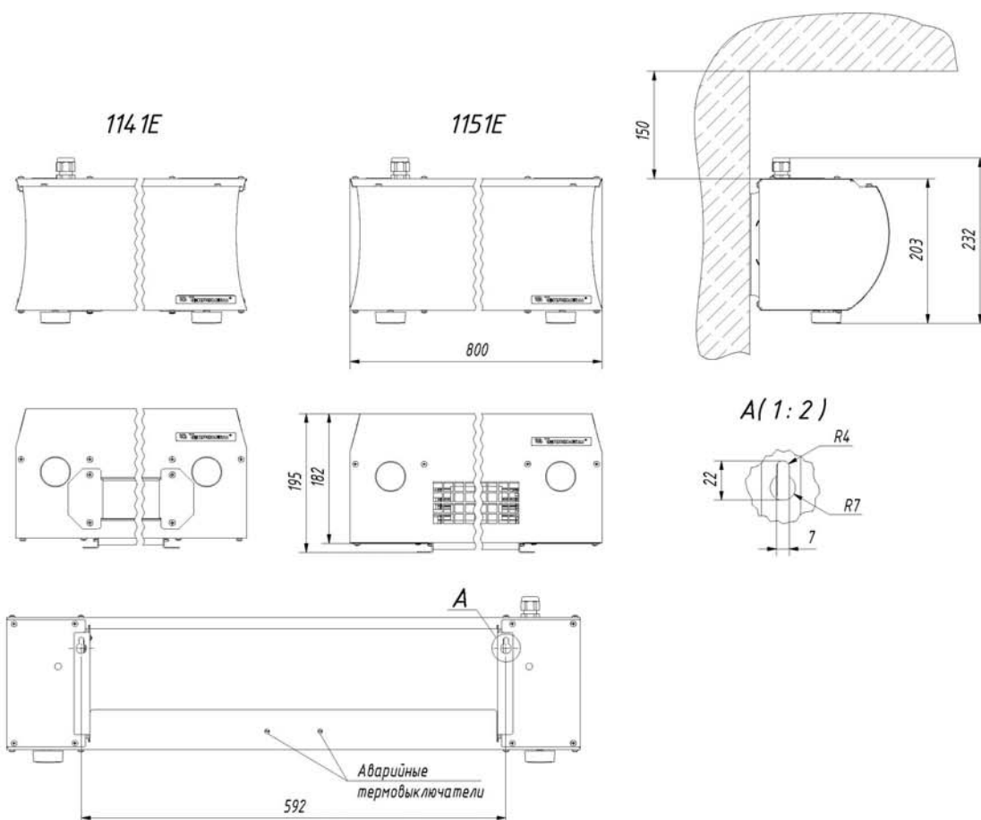
Рис. 7 Габаритные и крепежные размеры
