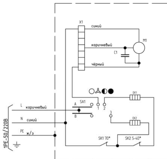
Рис. 5 Электрическая схема завесы КЭВ-4П1151Е
